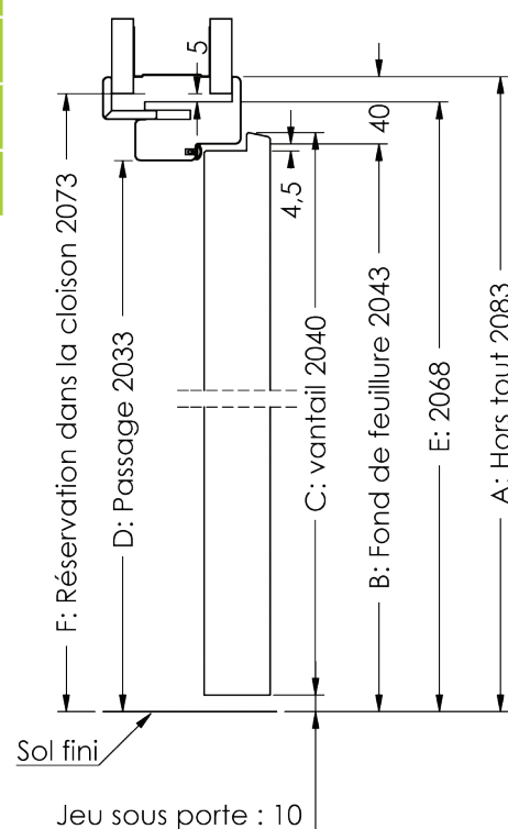
Coupe verticale
