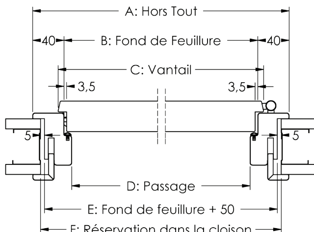
Coupe horizontale
